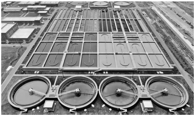
日前,由中铁十四局参建的天津市东丽区张贵庄污水处理厂二期工程通过竣工验收。该项目投用后日总处理污水量(一期与二期)可达45万吨,成为天津市处理能力最大的污水处理厂,对改善当地水环境具有重要作用。
